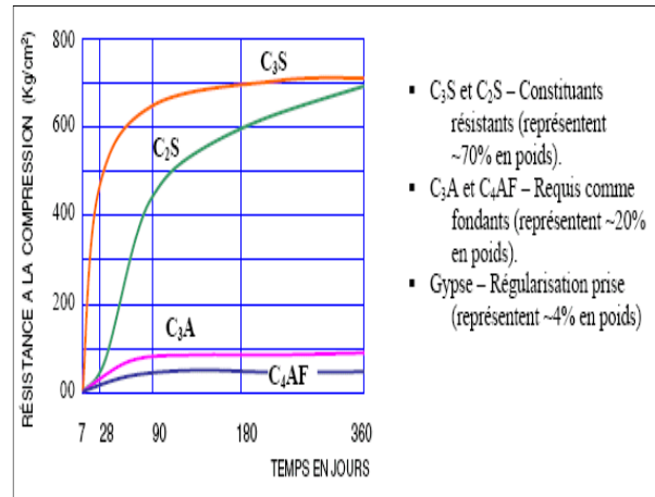
Figure. 3.13 (b): L'évolution des résistances des différents produits d'hydratation du ciment.
