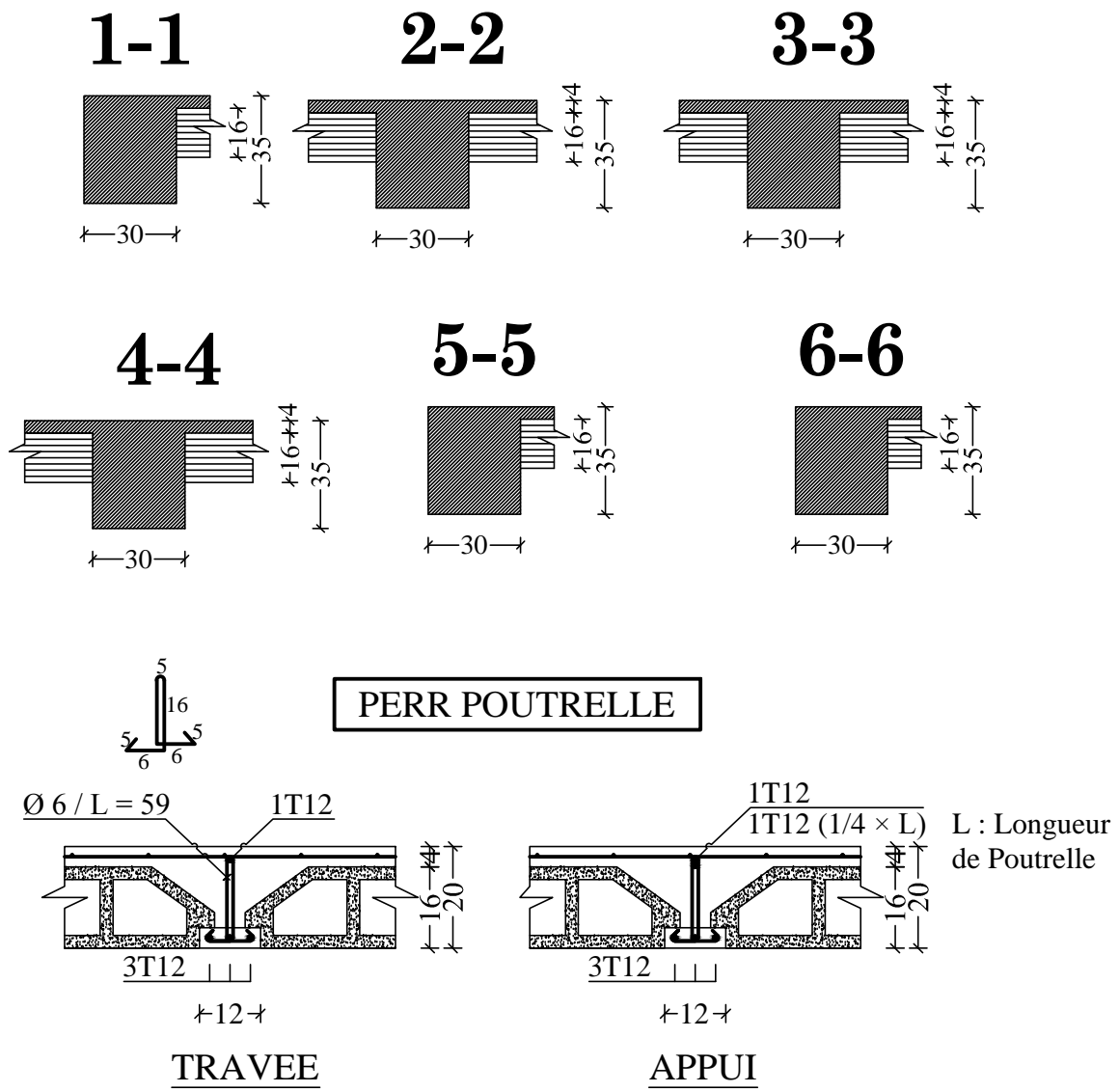
COFFRAGES ET FERRAILLAGES PLANCHER ECH:1/50-1/20
